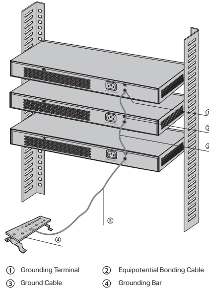
Figure 3-3 Equipotential Bonding
