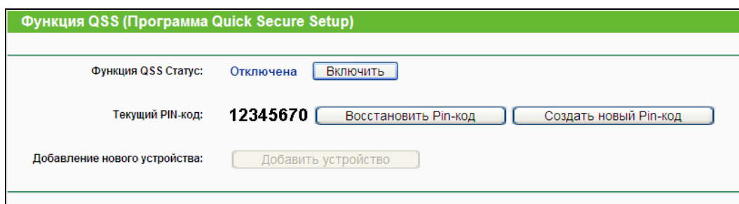
Рис. 4-2 Функция QSS
