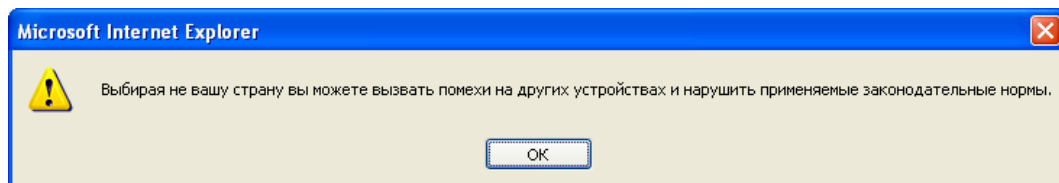
Информационное окно
