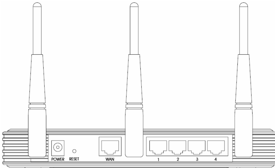
Рис. 1-2 Задняя панель
