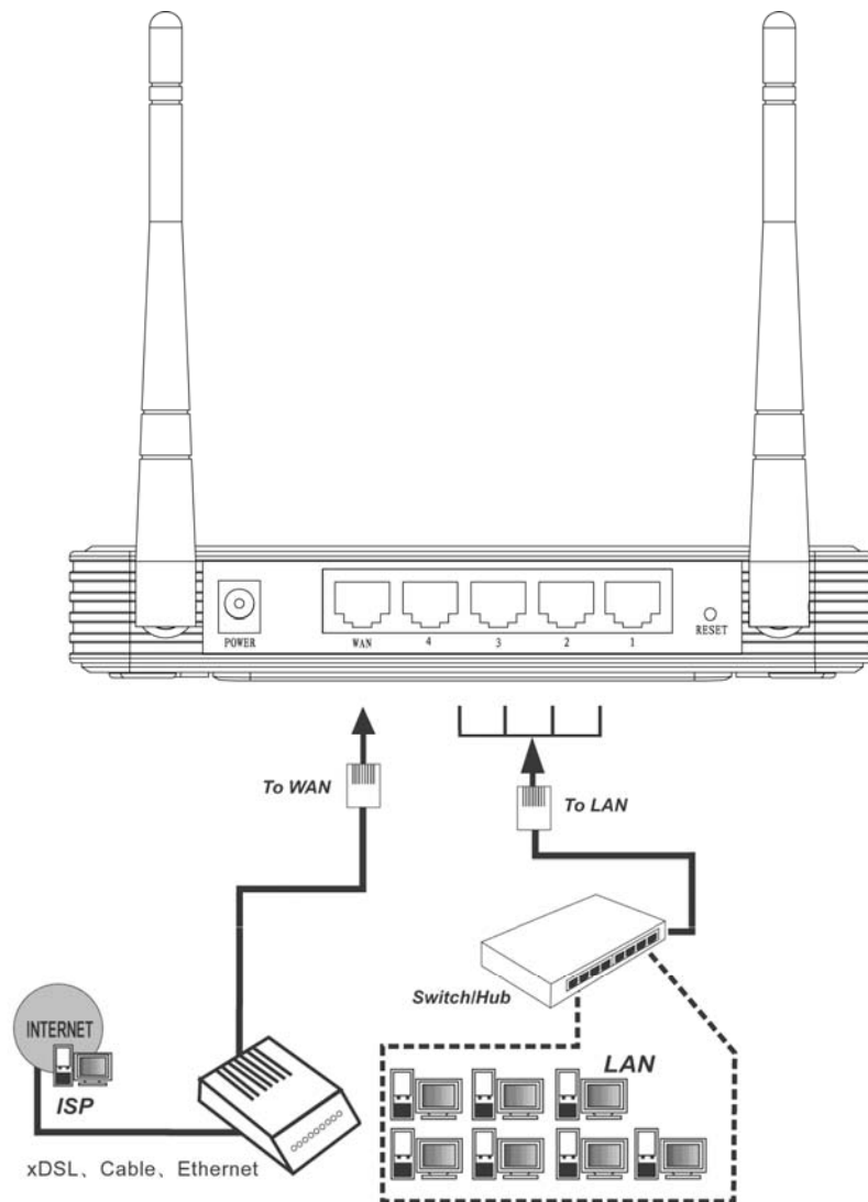
Bild 2-1 Hardwareinstallation des Routers
