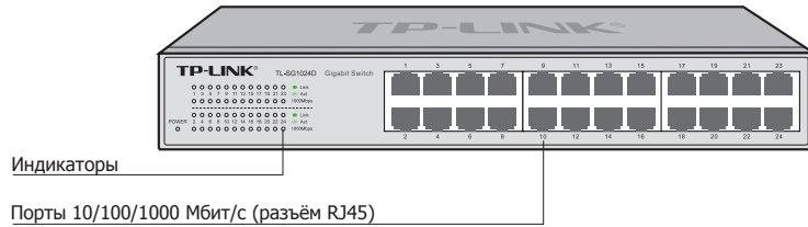
Рисунок 1-4 Передняя панель TL-SG1024D
