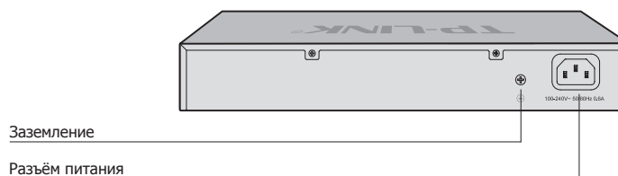
Рисунок 1-11 Задняя панель TL-SG1008
