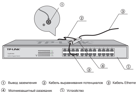
Рисунок 3-4 Выравнивание потенциалов
