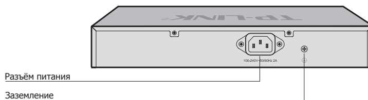
Рисунок 1-12 Задняя панель TL-SG1008PE
