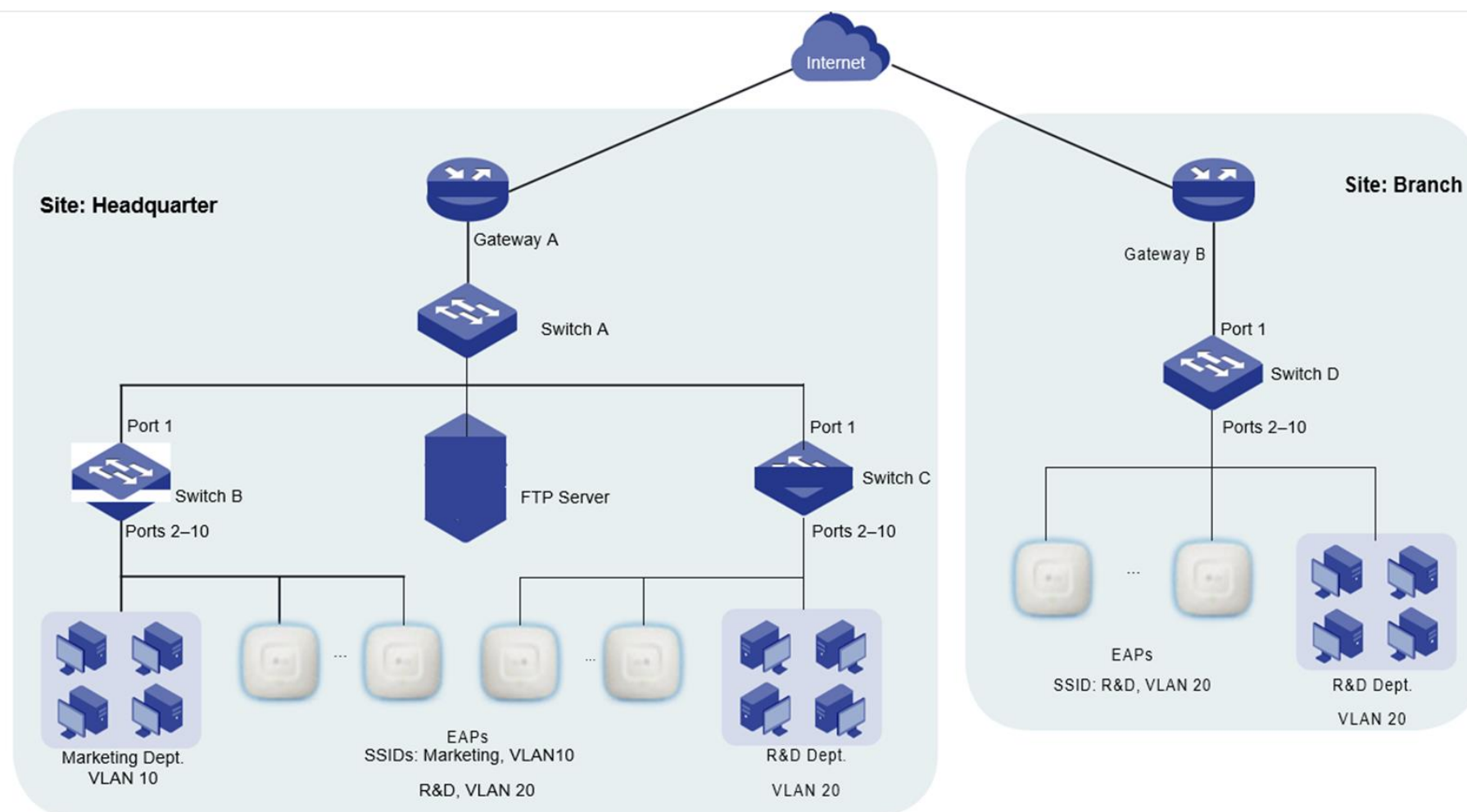
Topologie réseau Figure 2-2
