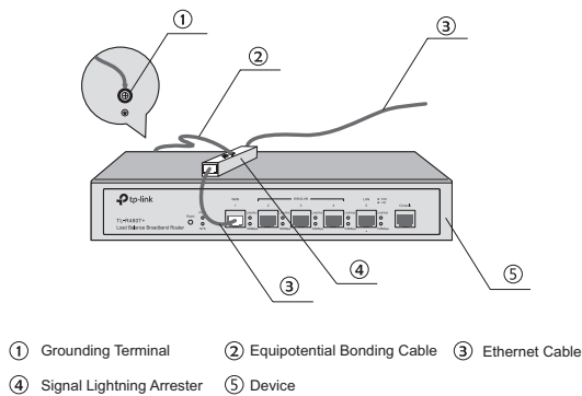
Figure 3-4 Equipotential Bonding
