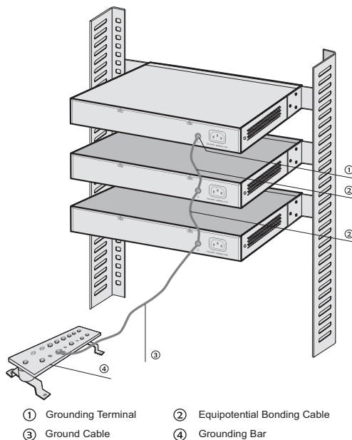
Figure 3-3 Equipotential Bonding
