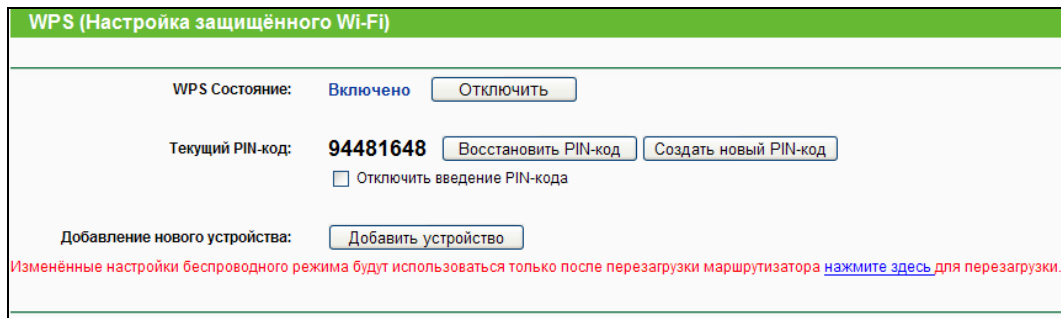
Рис. 4-16 Функция WPS
