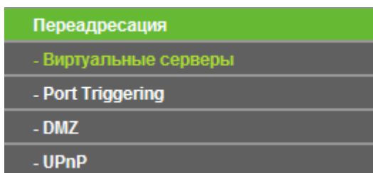
Рис. 4-62 Меню Переадресация
