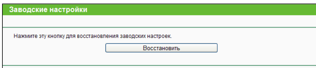
Рис. 4-121 Заводские настройки
