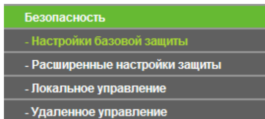
Рис. 4-69 Меню Безопасность
