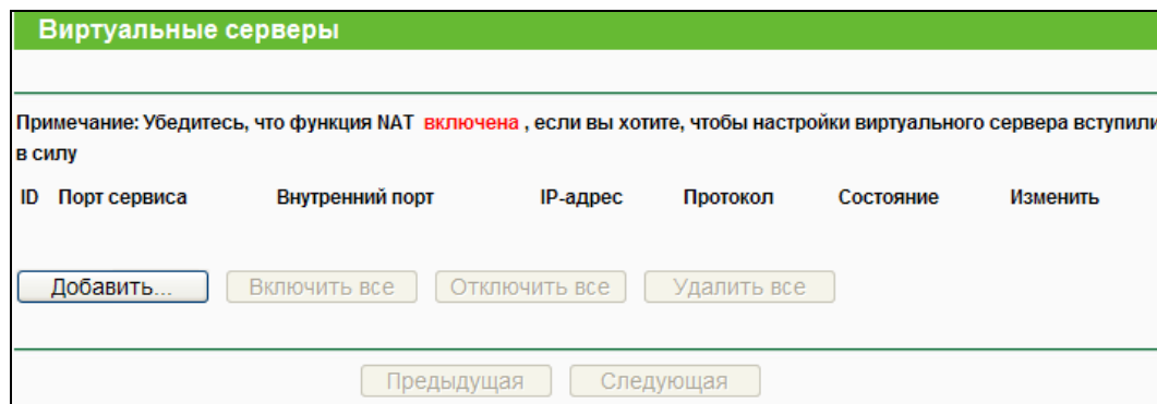
Рис. 4-63 Виртуальные серверы
