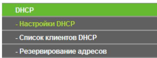
Рис. 4-42 Меню DHCP
