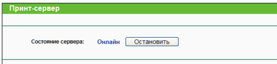
Рис 4-58 Настройка принт-сервера
