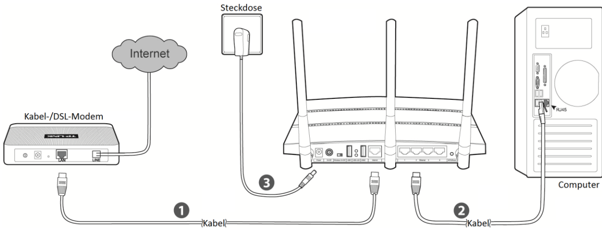
Bild 2-1 Hardwareinstallation
