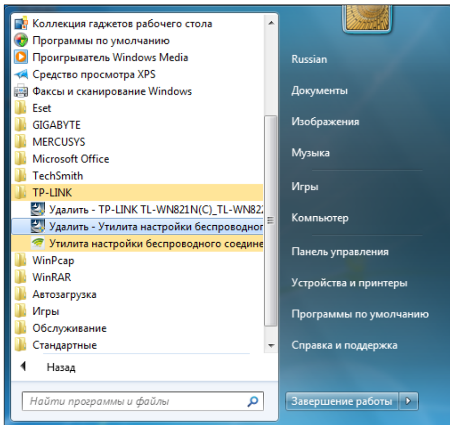
Рис. 6-1 Удаление утилиты
