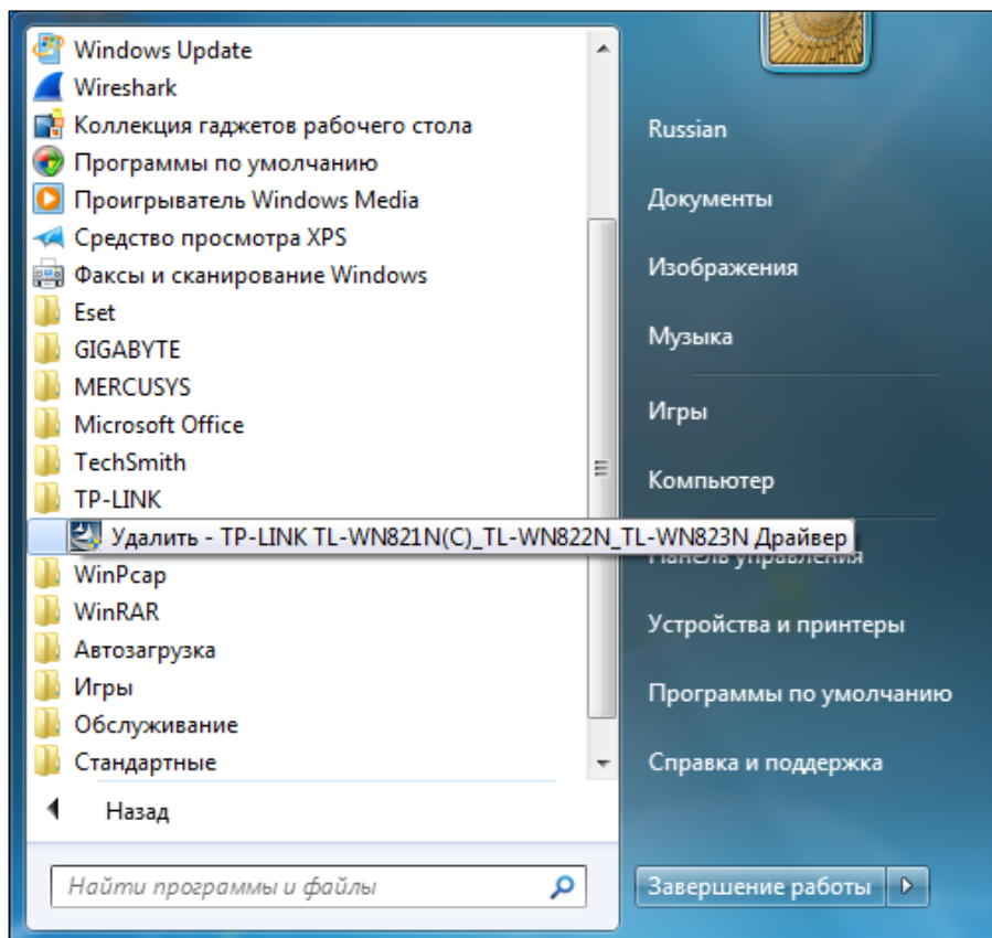
Рис. 6-4 Удаление драйверов
